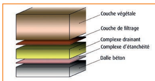
10 Coupe schématique des différentes couches de matériaux d'un passage végétalisé. Source : Cerema.
