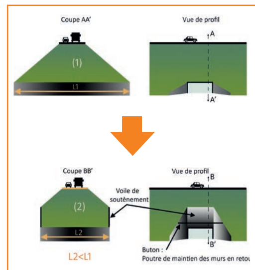
25 Représentation schématique d'un passage équipé d'un mur de soutènement vertical au-dessus de la tête d'ouvrage (2) et d'un passage non équipé (1). Source : Cerema.
