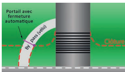
17 By-pass et portillon pour les vélos et piétons. Source : D. Chevalier, SETRA.
