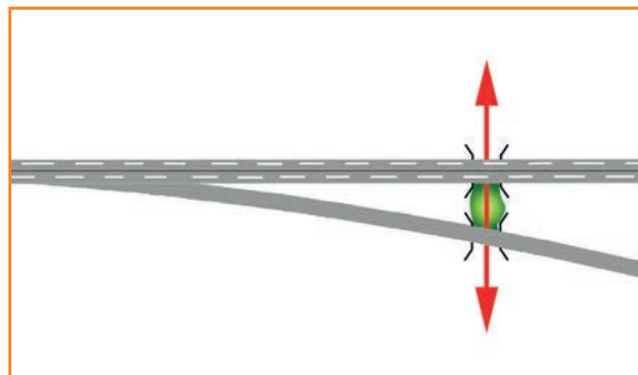
17 Représentation schématique du maintien de la continuité écologique au droit d'un échangeur par la réalisation de deux ouvrages successifs et la réalisation d'un cordon écologique entre les deux ouvrages. Source : Cerema.
