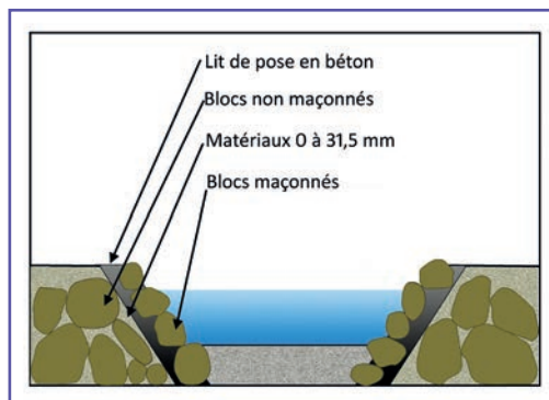
8 Schéma de principe de reconstitution des berges avec des blocs maçonnés. Source : Cerema.
