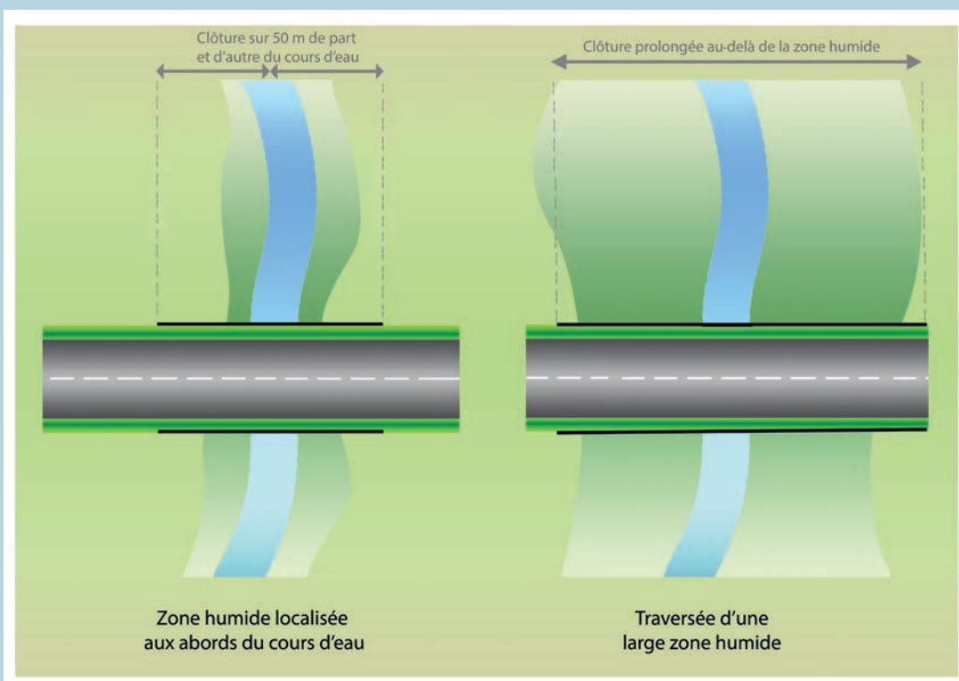
Schéma de principe d'implantation de clôtures pour le castor, le vison d'Europe et la loutre, à proximité d'un passage à faune dédié. Source : Cerema.
