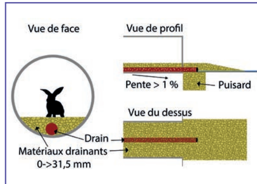
21 Schéma de principe de drainage d'un ouvrage pour maintenir au maximum le passage de la faune au sec. Source : Cerema.
