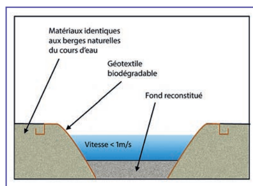
5 Schéma de principe de reconstitution des berges (et du pied sec) en matériaux identiques aux berges naturelles du cours d'eau. Source : Cerema.
