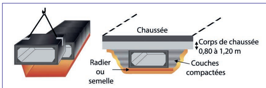
4 Schéma de principe d'un ouvrage cadre constitué d'une série d'éléments préfabriqués posés sur une semelle en béton maigre. Source : Cerema.
