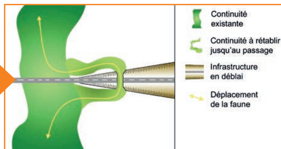
7 Décalage de l'ouvrage sur une section en déblai facilitant l'aménagement d'un passage. Source : Cerema.
