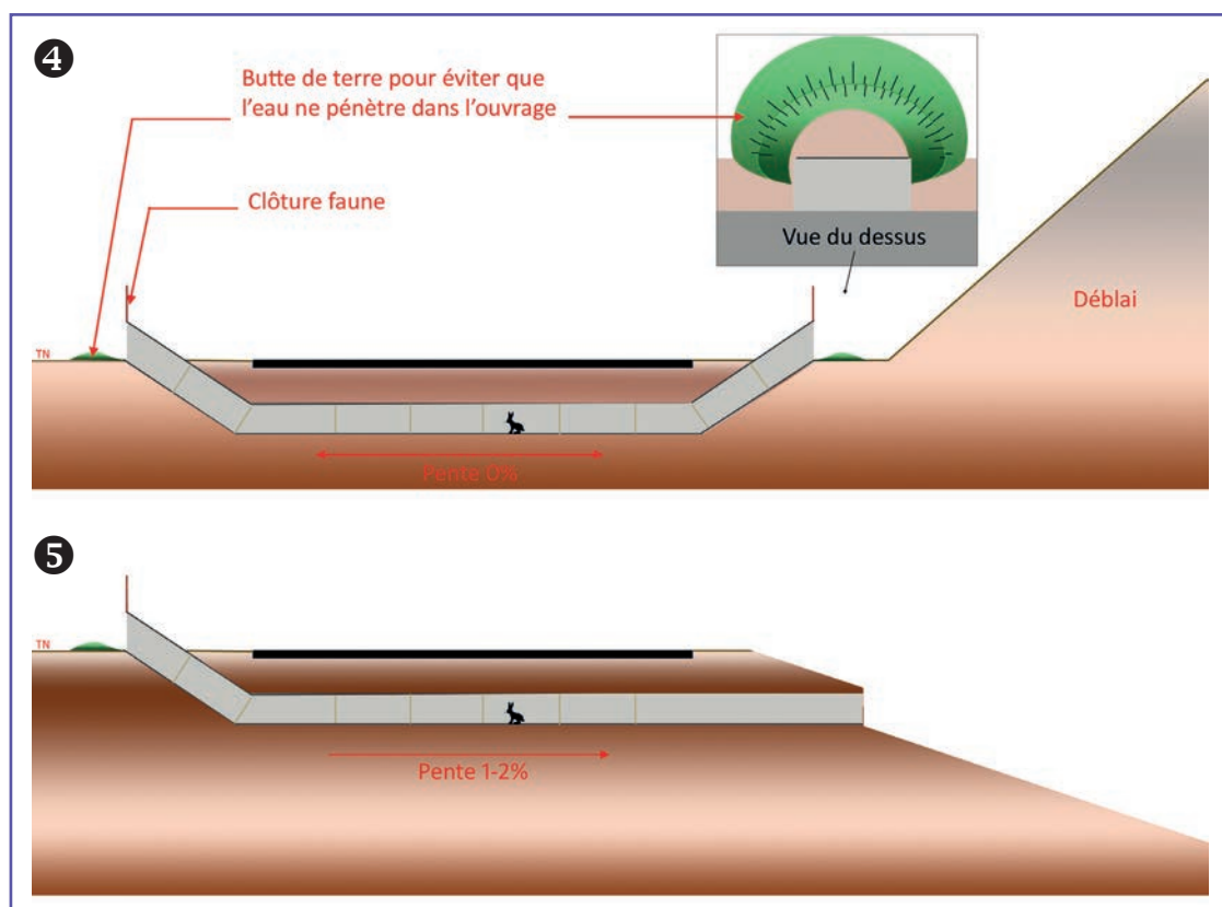
Profil en travers d'un passage petite faune présentant deux entrées en pente ❹ (ou une ❺) lorsque l'infrastructure est au niveau du terrain naturel. Source : Cerema.
