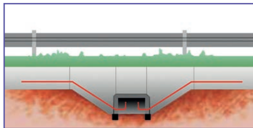
11 Schéma de principe d'une rampe d'accès au passage. Source : Cerema.
