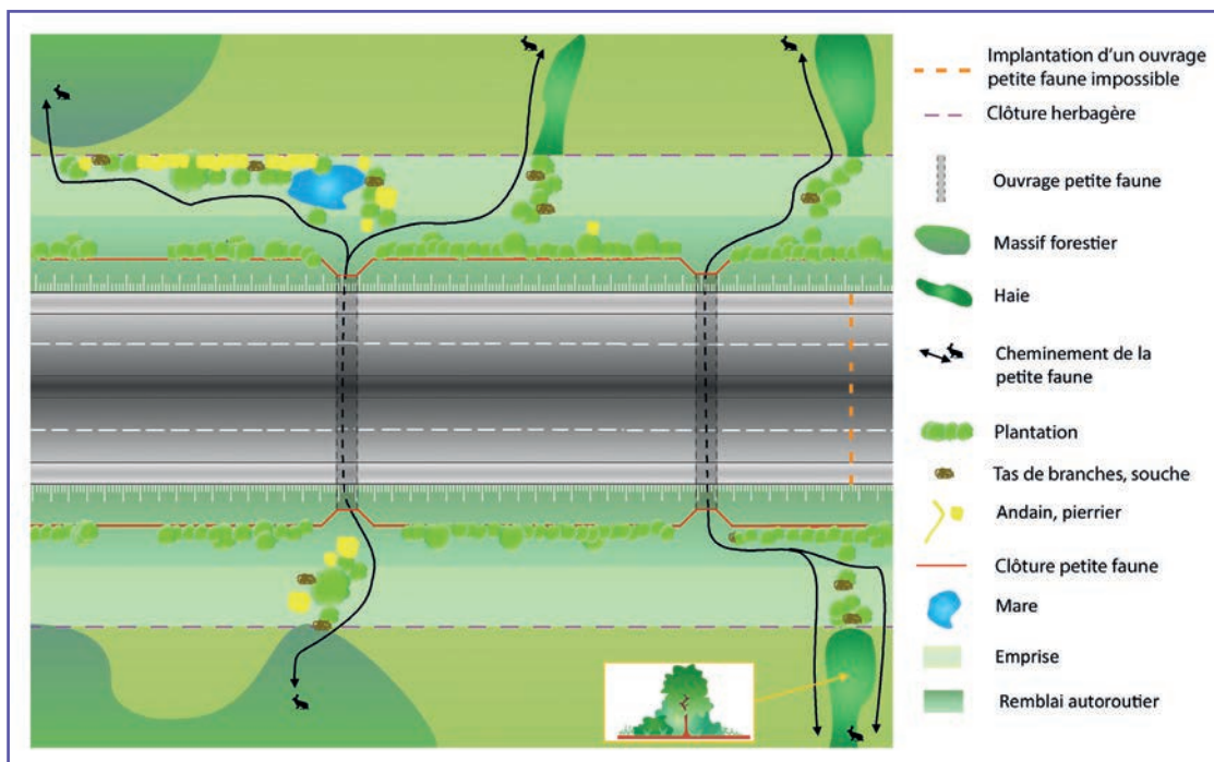
20 Principe de raccordement des ouvrages aux structures végétales existantes. Source : Cerema.
