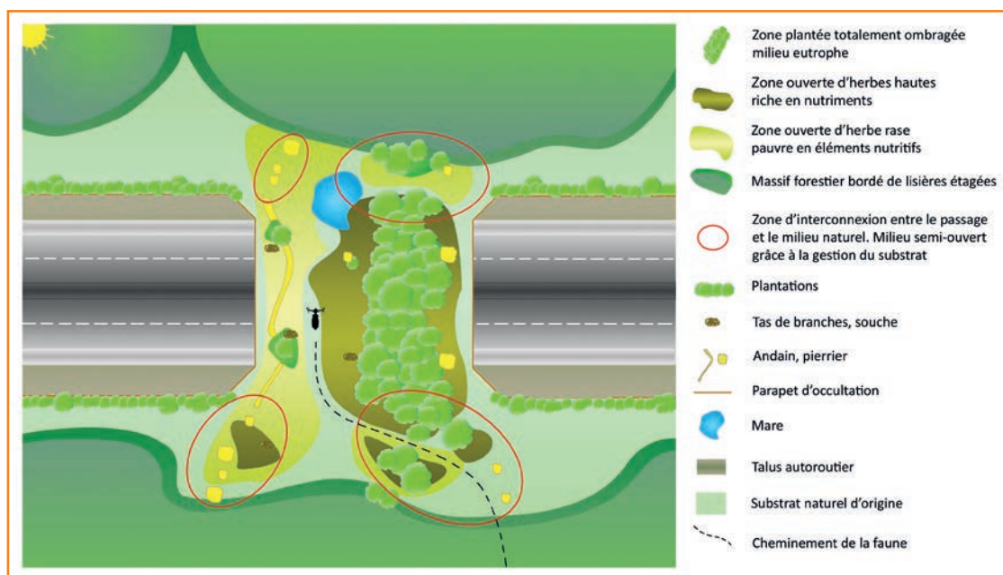
⑧ Exemple schématique d'aménagement d'un passage remarquable en contexte forestier. Source : Cerema, d'après BN Federal agency for Nature conservation, 2019.
