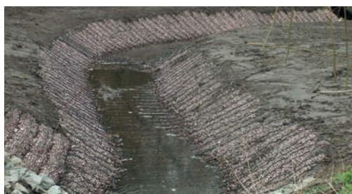
11 Reconstitution de berges en matelas de gabions*. Source : AquaTerra Solutions.
