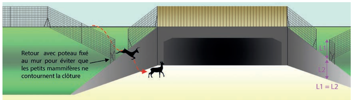
Exemple schématique de l'aménagement d'un système échappatoire au niveau des murs en aile d'un ouvrage inférieur. Source : Cerema.
