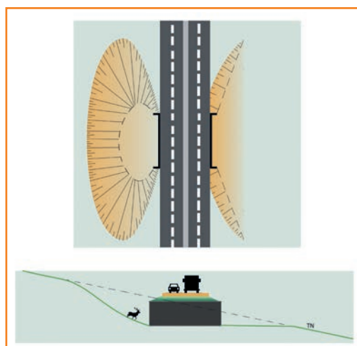
10 Vue schématique d'un passage inférieur en profil mixte avec fosse d'entonnement d'un côté. Source : Cerema.
