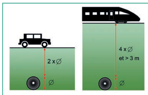
❶ Schéma représentant la hauteur de remblai à maintenir au-dessus de l'ouvrage en fonction du type d'infrastructure. Source : Cerema.
