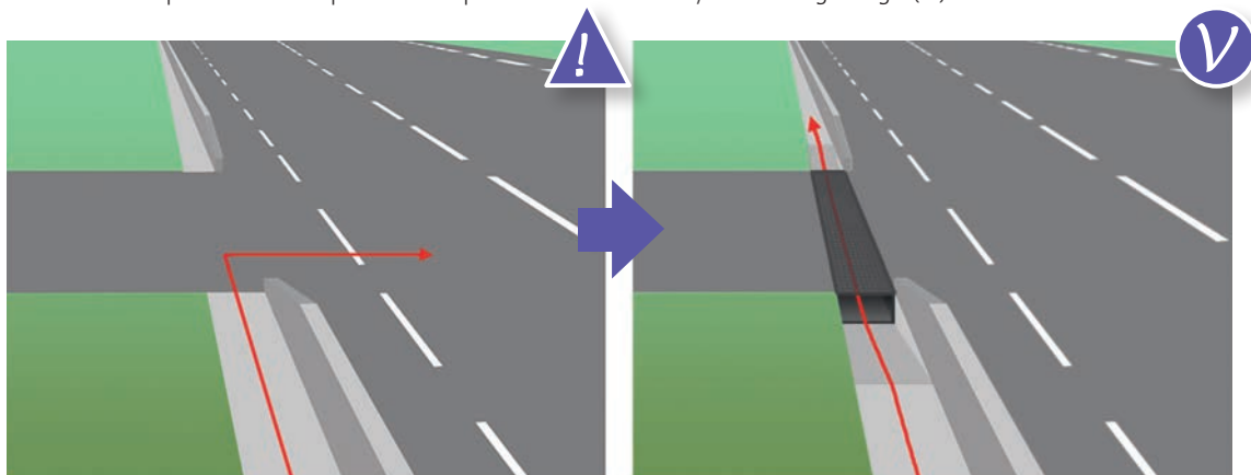
14 Dispositif de franchissement d'une voie perpendiculaire à l'infrastructure principale évitant aux amphibiens d'accéder à cette dernière. Source : Cerema.
