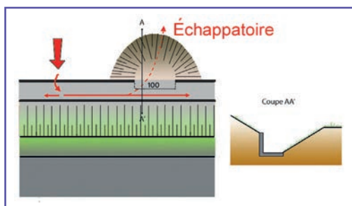
10 Schéma en plan d'un dispositif d'échappatoire. Source : Cerema.
