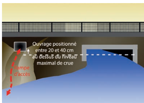
Schéma de principe de l'implantation d'un conduit sec à proximité d'un ouvrage hydraulique. Source : Cerema.
