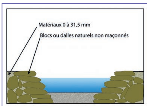
9 Schéma de principe de reconstitution des berges avec des blocs ou dalles naturels. Source : Cerema.
