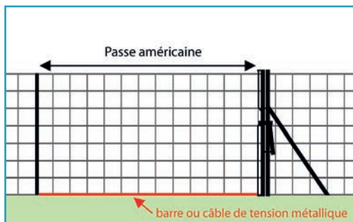
11 Représentation schématique d'une passe américaine équipée d'un câble ou d'une barre de tension métallique. Source : Cerema.
