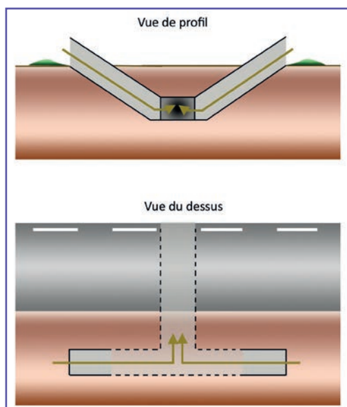
⑨ Schémas de principe d'un ouvrage dont l'entrée est parallèle à l'infrastructure et en pente jusqu'à atteindre la profondeur du passage sous l'infrastructure. Source : Cerema.
