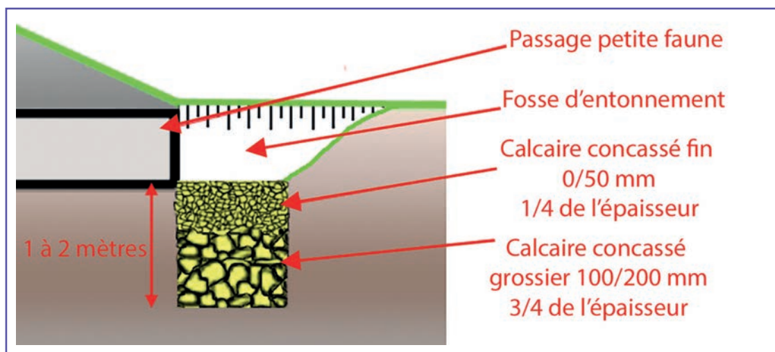
⑪ Principe de fosse de drainage à l'entrée d'un passage petite faune. Source : Cerema.
