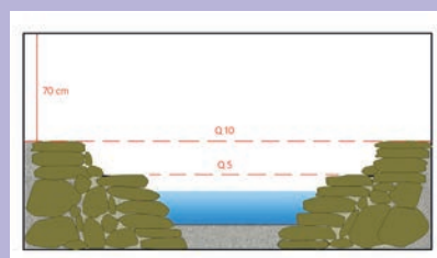
Schéma de principe d'une banquette en gradins. Source : Cerema.
