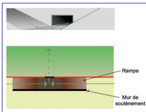
6 Schéma de principe d'une rampe d'accès au passage petite faune. Source : Cerema.
