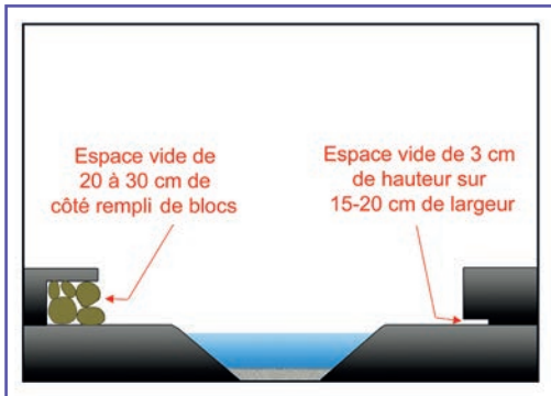
16 Schéma de principe de création d'abris au sein des banquettes faune. Source : Cerema.
