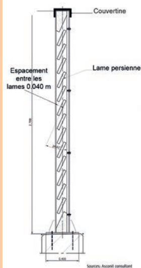
DETAIL EN COUPE D'UNE PALISSADE OCCULTANTE AVEC SYSTEME DE LAMES EN BOIS AJOURÉES
