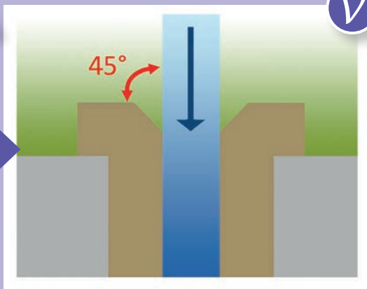
16 Schéma de principe d'aménagement de la banquette petite faune à l'entrée d'un ouvrage pour éviter l'érosion des berges. Source : Cerema.
