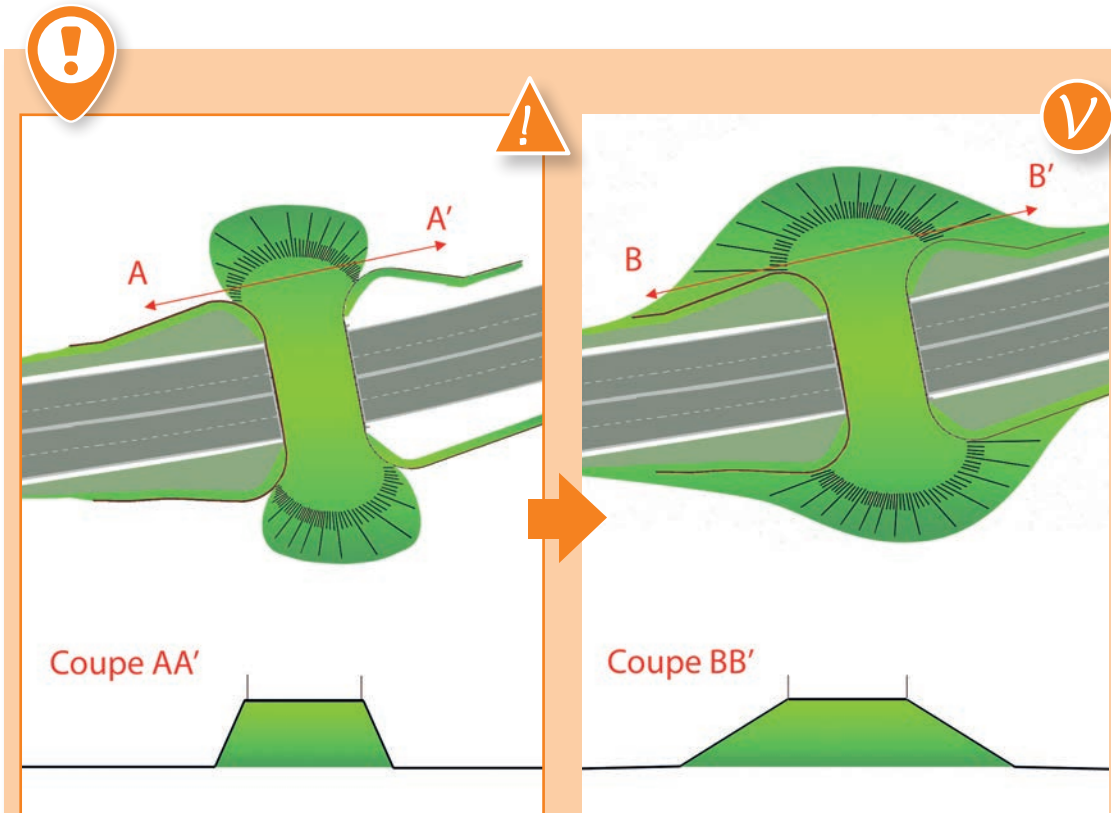
④ Les rampes d'accès doivent être en pente douce quelle que soit la direction. Source : Cerema.
