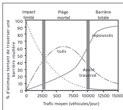
Effet de fragmentation des infrastructures routières en fonction du trafic moyen journalier. Source : Rapport COST 341 adapté de Seiler, 2003.
