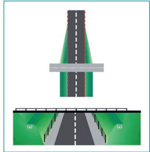
(3) Perré de l'ouvrage maintenu franchissable par la faune en positionnant la clôture en bas du perré et en créant des faux plats dans le perré (a).
