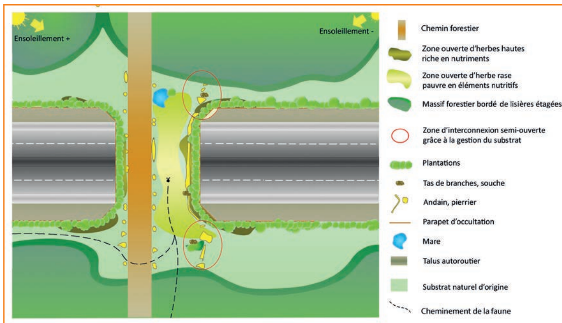
6 Exemple schématique d'aménagement d'un passage supérieur ordinaire mixte en contexte forestier. Source : Cerema.
