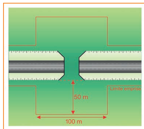
(26) Exemple schématique d'une surface d'aménagement de 5 000 m 2 à réserver aux abords d'un passage toute faune exceptionnel. Source : Cerema.
