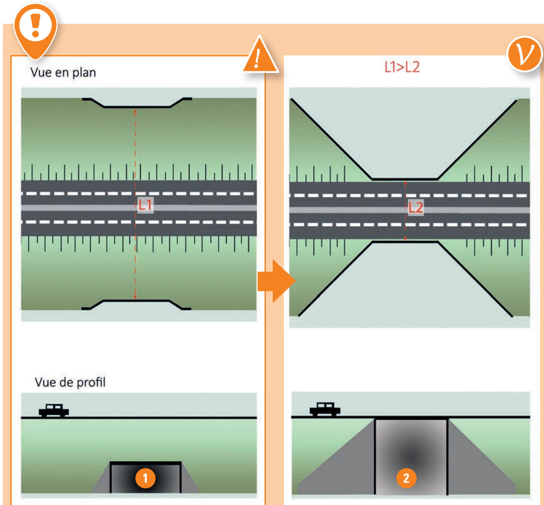
23 Représentation schématique d'un passage avec un remblai au-dessus du tablier (1) et d'un ouvrage d'une hauteur équivalente au remblai (2). Source : Cerema.
