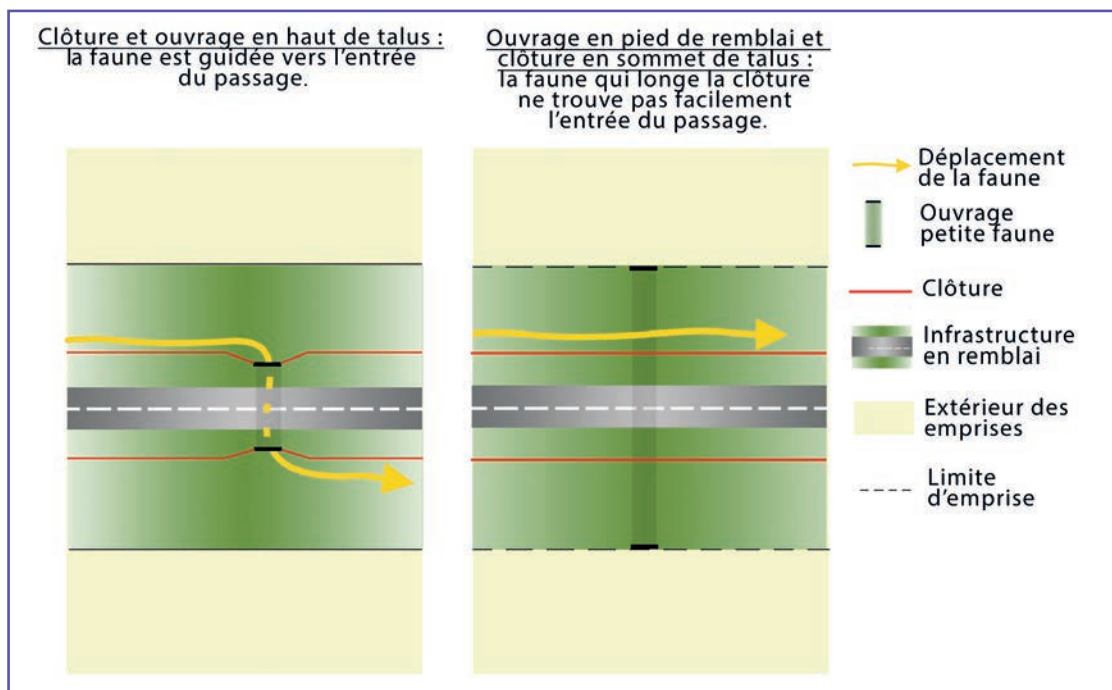
❷ Schéma de principe permettant de visualiser l'intérêt de positionner à la fois les clôtures et les passages petite faune en haut de talus. Source : Cerema.
