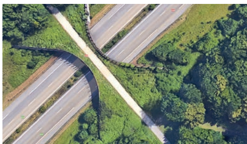
❷ Passage supérieur mixte ordinaire toute faune. Autoroute A36 (Région Grand Est). Source : Google Earth.
