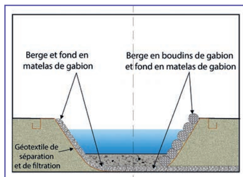
10 Schéma de principe de reconstitution des berges avec des boudins de gabions*. Source : Cerema.
