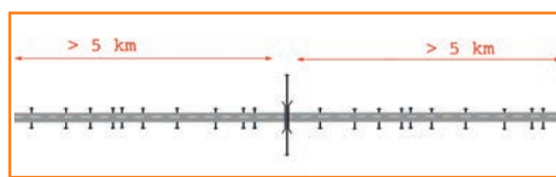
3 Représentation schématique de l'implantation d'un passage toute faune sur une section d'infrastructure équipée de passages petite faune et ne présentant pas d'enjeu fort.
