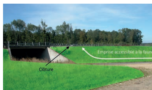
Clôture positionnée au plus proche de la route et permettant le libre accès des dépendances vertes à la faune. Source : Cerema.
