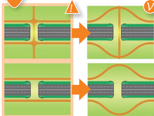
18 Schéma de principe du positionnement d'un chemin agricole ou forestier aux abords d'un passage faune. Source : Cerema.
