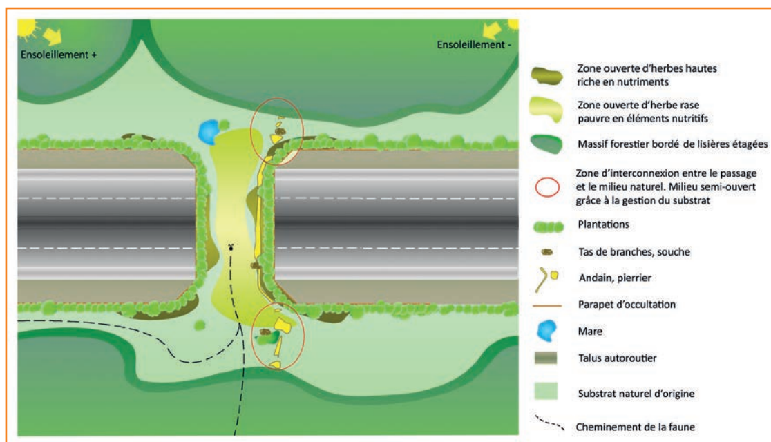
5 Exemple schématique d'aménagement d'un passage supérieur ordinaire en contexte forestier. Source : Cerema.
