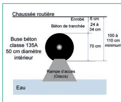
Principe d'implantation d'une buse sous chaussée. Source : PNR du Marais Poitevin. François Varenne - LPO 85.
