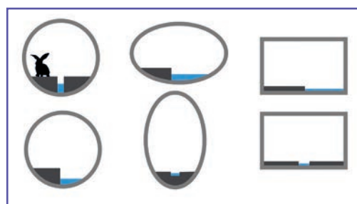
19 Schéma de principe de dispositifs de concentration des faibles écoulements dans un ouvrage. Source : Cerema.
