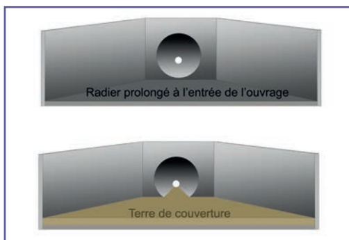
18 Schéma de principe d'un radier au sortir de l'ouvrage. Source : Cerema.
