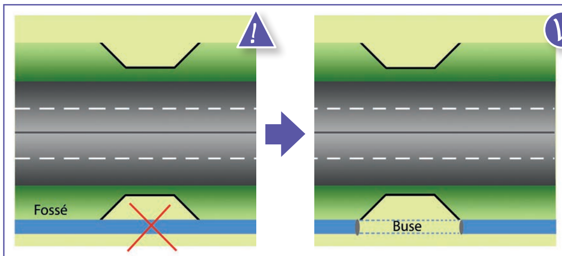
13 Schéma de principe d'installation d'une buse pour supprimer l'obstacle créé par un fossé situé au sortir d'un passage petite faune. Source : Cerema.
