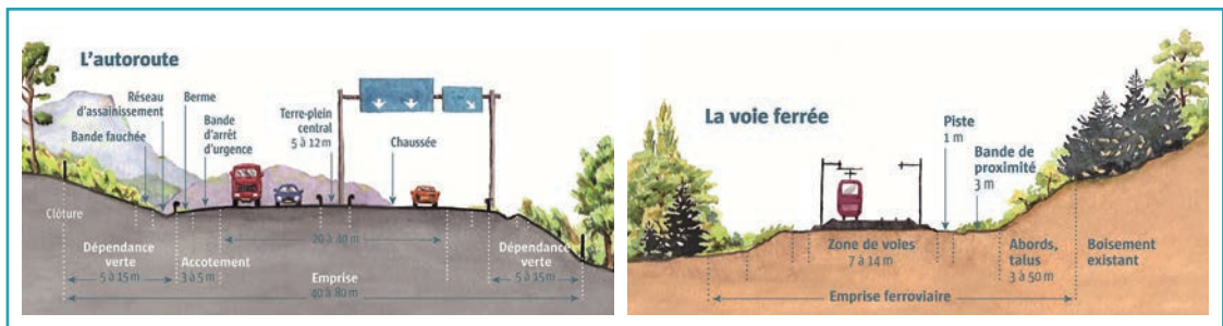
Profil en travers d'une autoroute et d'une voie ferrée.
