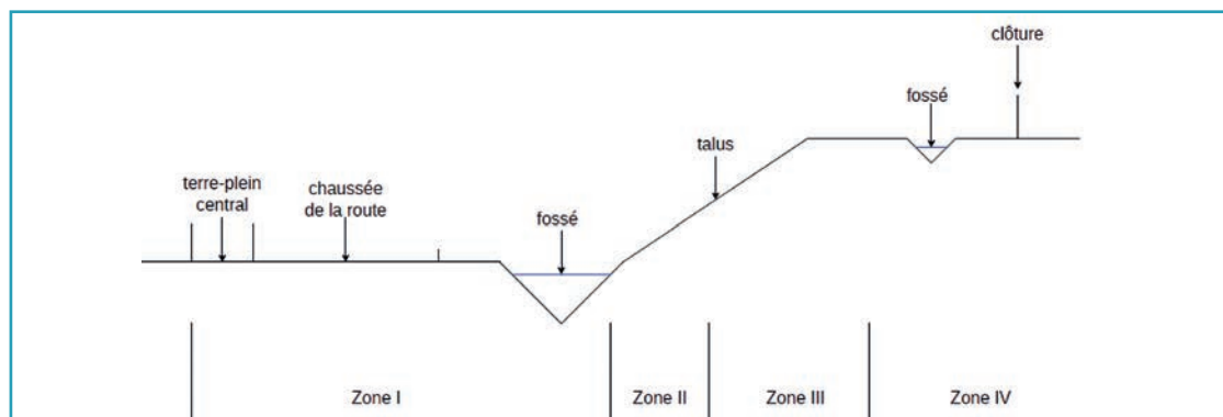
⑥ Coupe schématique d'une dépendance verte d'une infrastructure routière. Source : Cerema.
