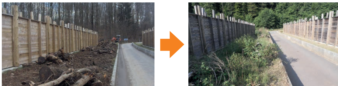
15 Aménagement d'un amas de branches en phase travaux et son évolution deux ans après. RD64 (70). Source : Jean-Paul Chatel. DIR Est.
