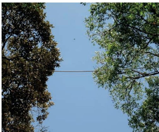
Corridor équipé d'un pont de singe pour rétablir la liaison en canopée (RN2 - Guyane). Source : Cerema.
