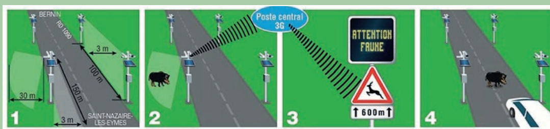
4 Vue schématique du détecteur de faune. Source : Conseil départemental de l'Isère.
