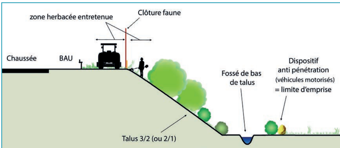
1 Position de la clôture en haut de talus permettant d'intégrer les dépendances vertes aux habitats d'espèces et d'assurer une continuité longitudinale naturelle. Source : Cerema.
