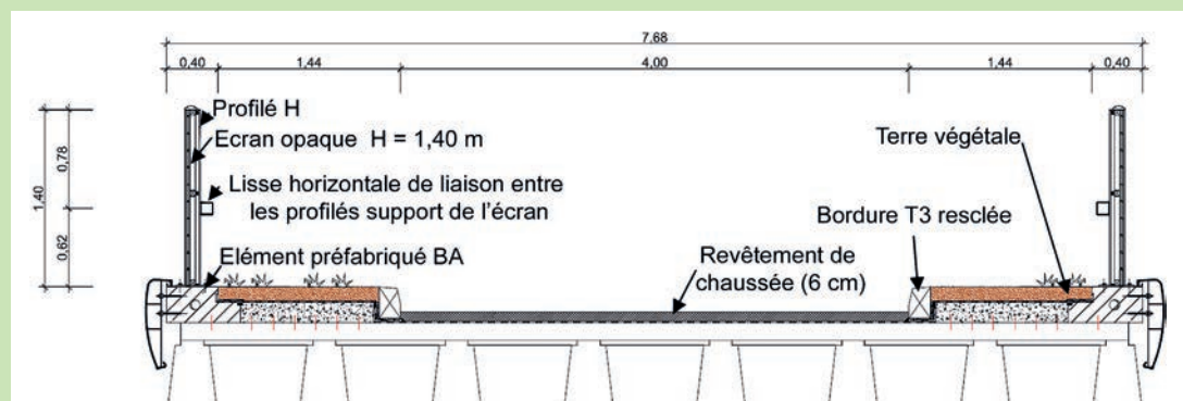
Schéma de principe de l'aménagement. Source : Vinci Autoroutes - Cofiroute.
