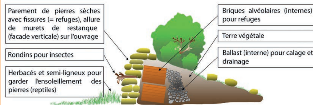
Mise en œuvre des écorestanques « en série ». Autoroutes A8 et A57. Source : C. Buton, Cabinet X-Aequo.
