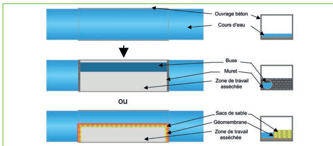
⑧ Principe de dévoiement provisoire d'un cours d'eau pour effectuer des travaux à l'intérieur d'un ouvrage. Source : Cerema.
