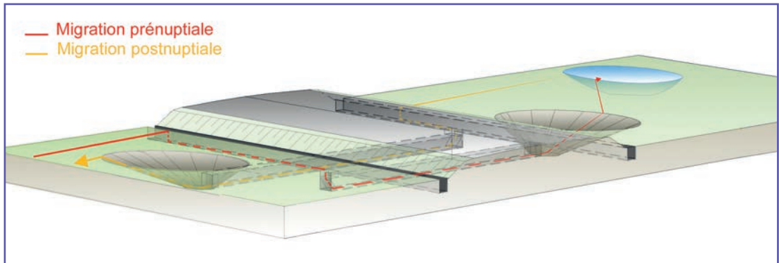
⑥ Représentation schématique d'un dispositif de franchissement à sens unique et du cheminement des amphibiens suivant le sens de leur déplacement. Source : Cerema.
