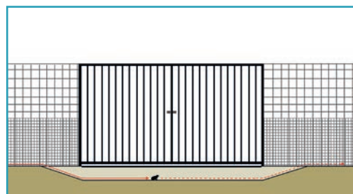
7 Schéma d'implantation d'un caniveau au droit d'un portail. Source : Cerema.
