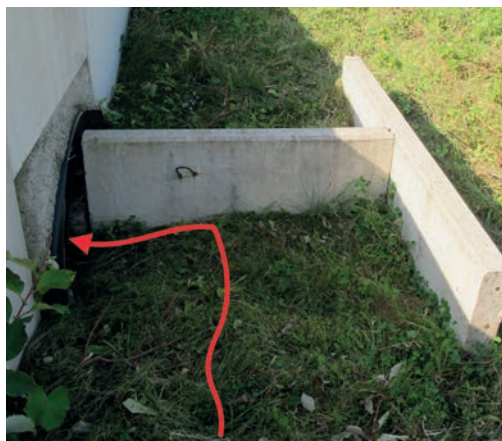
13 Dispositif de guidage visant à faciliter l'utilisation du passage par les amphibiens. Source : Cerema.
