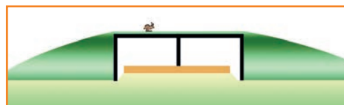
❷ Représentation schématique d'un ouvrage réalisé sur une infrastructure située au niveau du terrain naturel et nécessitant des rampes d'accès pour la faune. Source : Cerema.
