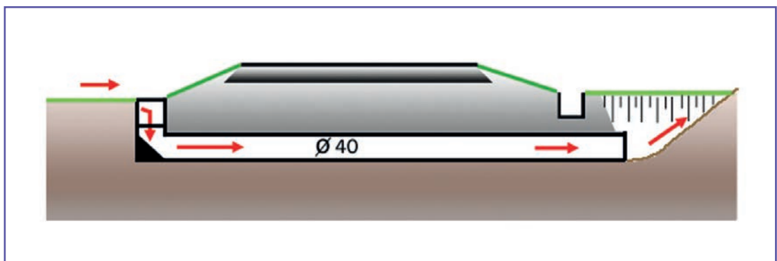
⑨ Profil en travers d'un conduit à sens unique. Source : Cerema.
