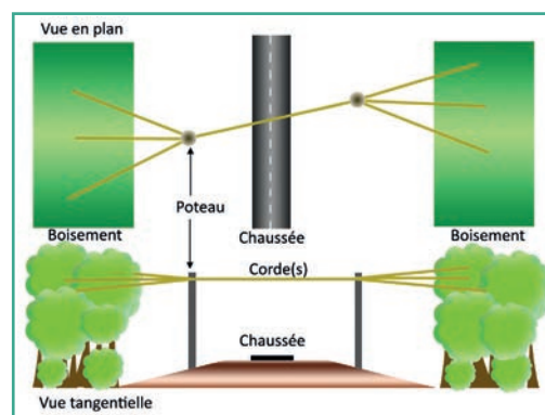
② Schéma de principe d'un corridor par canopée. Source : Cerema.
