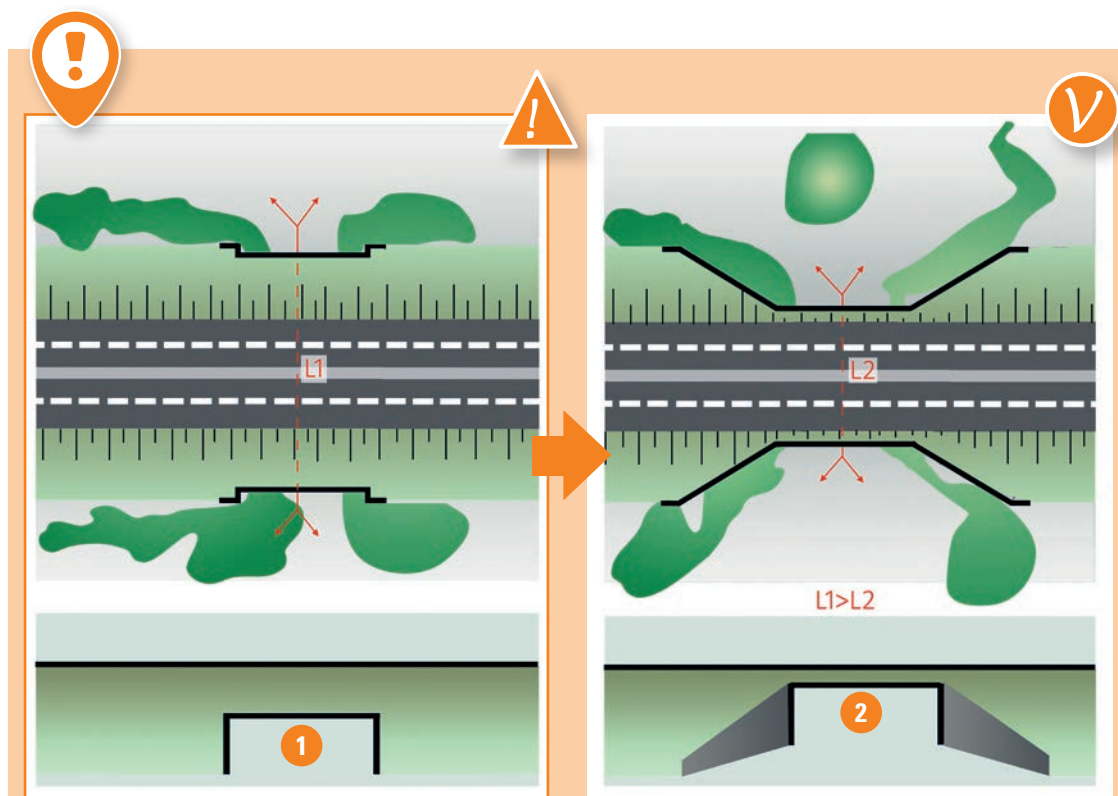
21 Représentation schématique d'un ouvrage sans (1) et avec (2) murs de soutènement en « aile ». La longueur de traversée est réduite lorsque l'ouvrage en est équipé. Source : Cerema.
