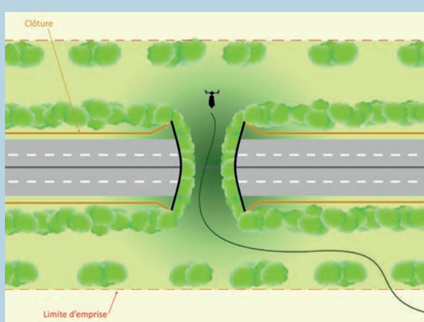
Schéma de principe d'une double haie. Source : Cerema.
