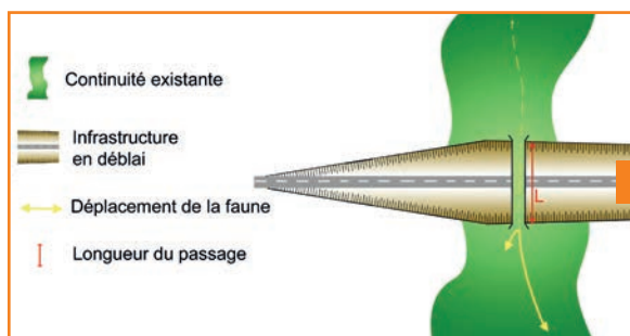
8 Infrastructure en fort déblai induisant une grande longueur de traversée sur le passage. Source : Cerema.
