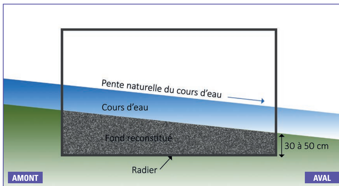
② Schéma de principe d'implantation d'un ouvrage hydraulique avec radier. Source : Cerema.
