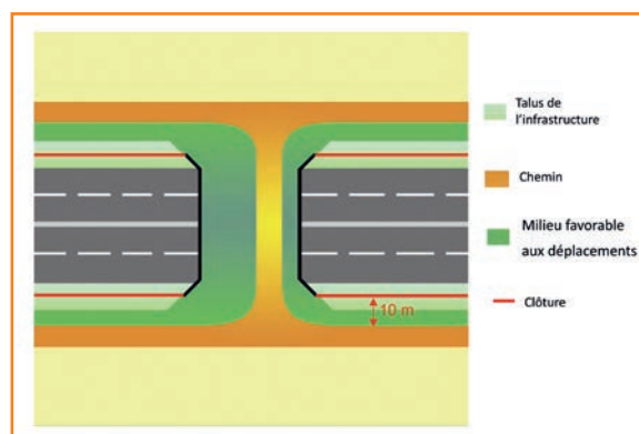
19 Schéma de principe du maintien d'un couloir naturel de 10 m entre le chemin longeant l'infrastructure et la clôture. Source : Cerema.
