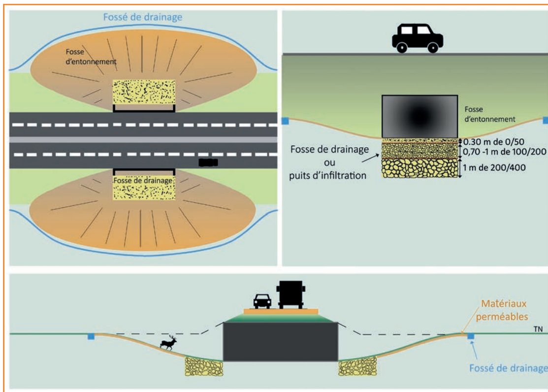
9 Schémas de l'aménagement d'une fosse de drainage sur les passages inférieurs situés sous le niveau du terrain naturel. Source : Cerema.
