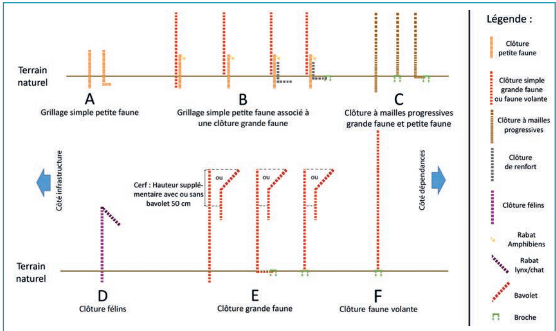
Schéma de l'ensemble des catégories de clôtures. Source : Cerema.
