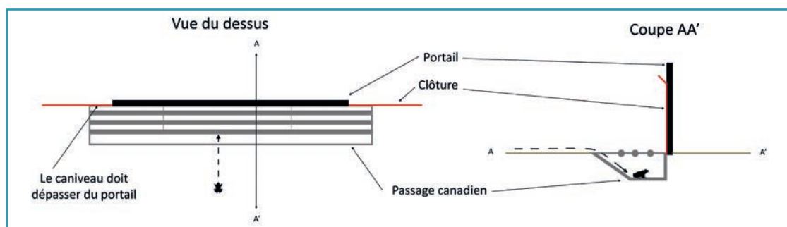
9 Représentation schématique d'un dispositif de passage canadien équipé d'une rampe pour empêcher l'accès des amphibiens. Source : Cerema.
