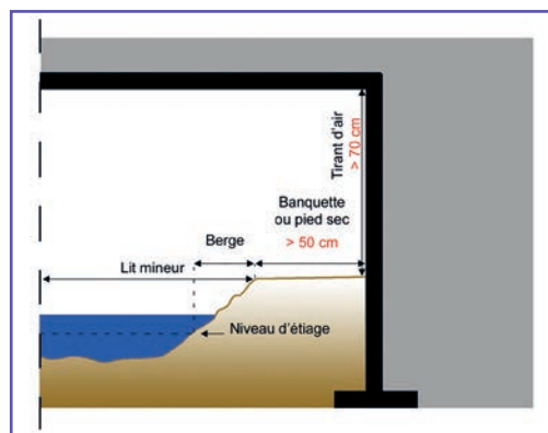
3 Schéma de principe d'une banquette petite faune dans un ouvrage hydraulique. Source : Cerema.
