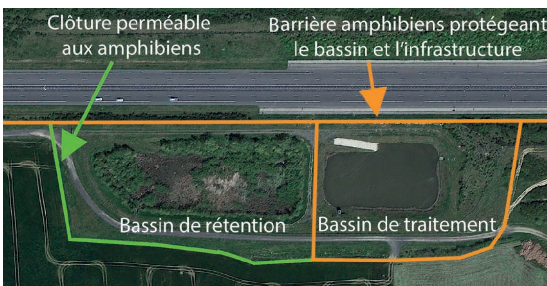
(19) RN 59 section Saint-Clément Azerailles. À droite sur la photo, le bassin de traitement est clôturé pour être inaccessible aux amphibiens, alors que le bassin de rétention situé à gauche de l'image leur est accessible (clôture perméable aux amphibiens). Source : Cerema.
