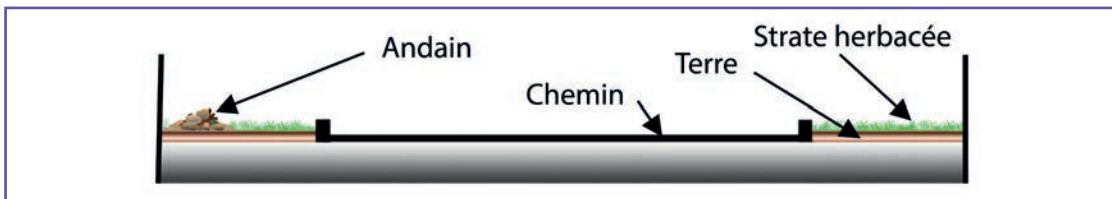
❸ Schéma de principe de l'aménagement de bandes enherbées sur un passage supérieur. Source : Cerema.
