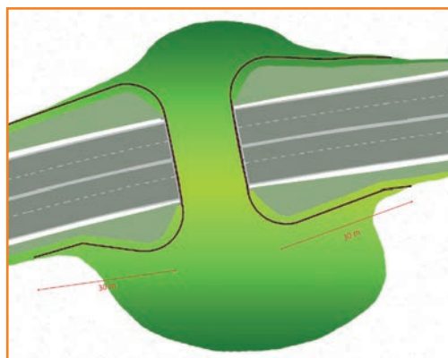
33 Schéma de principe de l'implantation d'un parapet d'occultation aux entrées d'un passage supérieur à faune. Source : Cerema.
