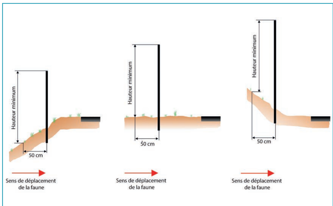
Détermination de la hauteur minimale de la clôture selon la configuration du terrain.
