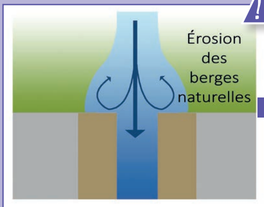
15 Schéma de principe d'une banquette petite faune risquant de favoriser l'érosion des berges à l'entrée de l'ouvrage. Source : Cerema.
