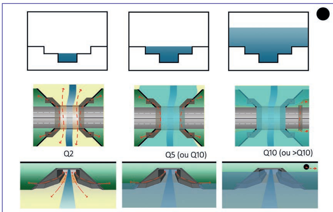
④ Schéma représentatif des possibilités de franchissement d'un ouvrage équipé d'une banquette petite faune en gradins à différents niveaux de débit. Source : Cerema.
