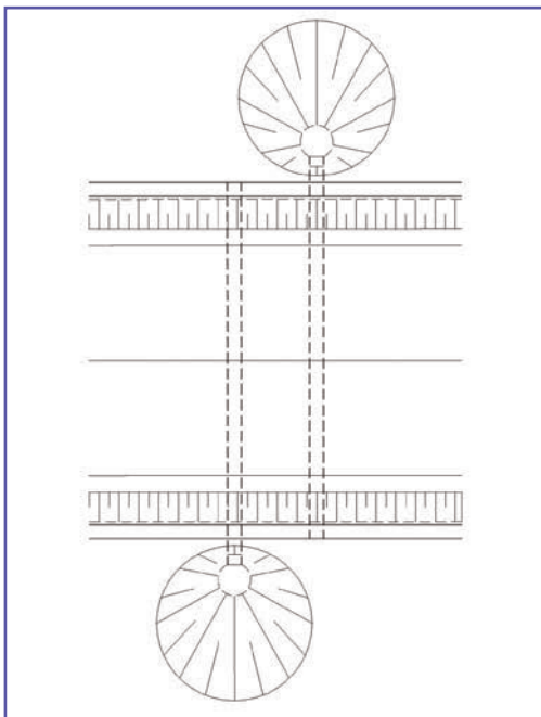
⑦ Vue en plan d'un double conduit. Source : Cerema.
