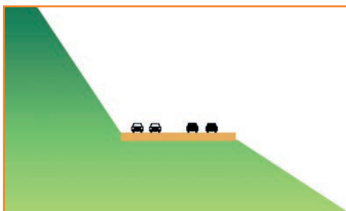
5 Exemple schématique d'un profil mixte marqué où l'insertion d'un ouvrage est complexe. Source : Cerema.
