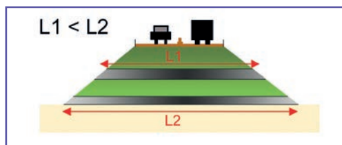
❶ Schéma de principe de l'implantation d'un ouvrage petite faune dans un remblai. L'ouvrage doit être positionné au plus haut dans le remblai pour limiter la longueur de traversée. Source : Cerema.
